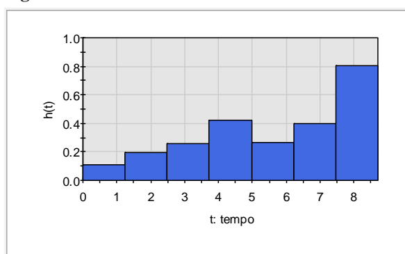
Figura 2 - Taxa de Falha.
