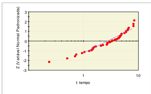
Figura 5 – Papel de probabilidade para a distribuição lognormal.
