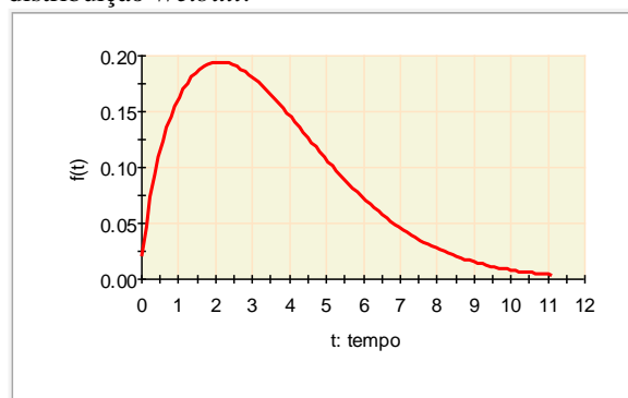
Figura 3 - Função densidade de probabilidade da distribuição Weibull .
