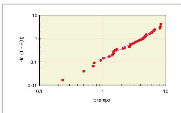
Figura 6 – Papel de probabilidade para a distribuição Weibull.
