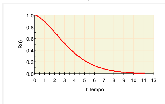
Figura 8 – Gráfico da função Confiabilidade R(t) .
